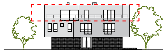
SJEVEROISTOČNA FASADA
